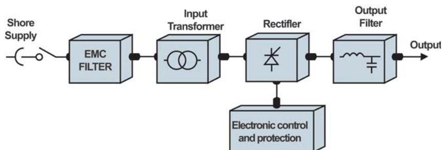
Battery Charger Circuit Circuitazione Caricabatteria
